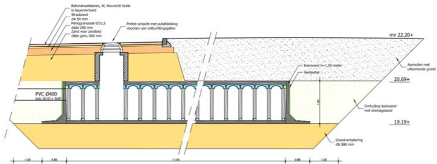
Figuur 2: Infiltratiekelder Don Boscostraat (tekening B1361R, Janssen de Jong)
